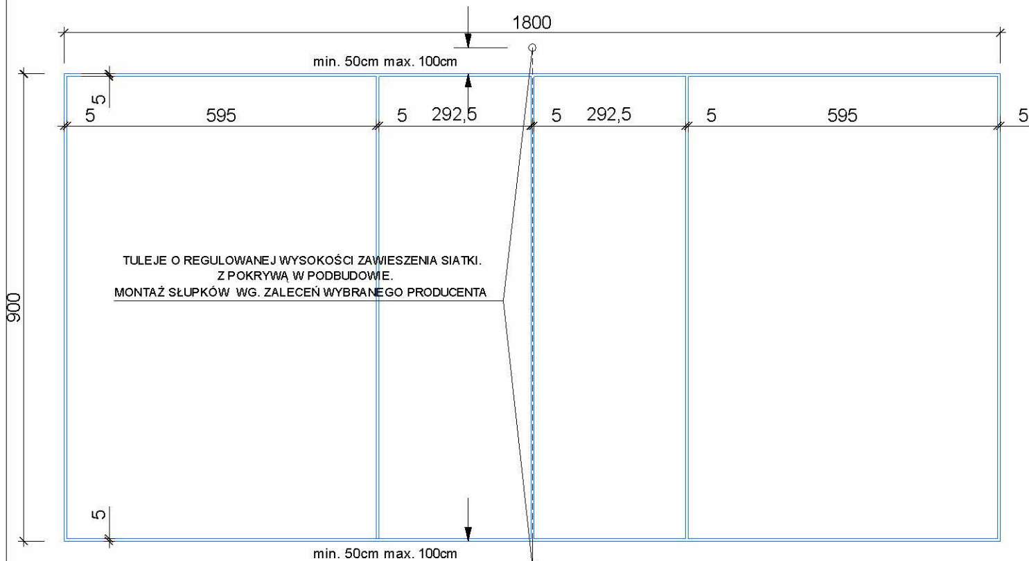
SŁUPEK DO SIATKÓWKI
